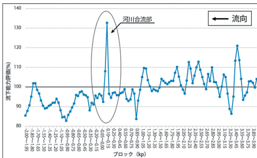
図3 流下能力の評価結果
