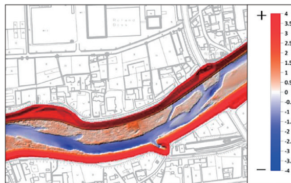
図5 河床高表現図
