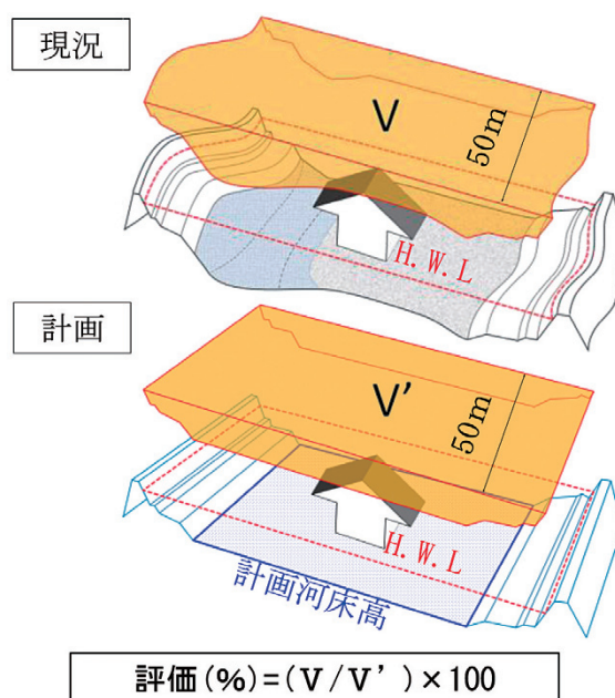
図2 流下能力の評価方法
